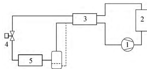
1 压缩机; 2 气体冷却器; 3 回热器; 4 节流阀; 5 蒸发器
