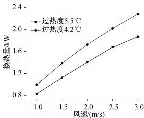
图2 过热度和风速对CO 2 蒸发器换热量的影响
